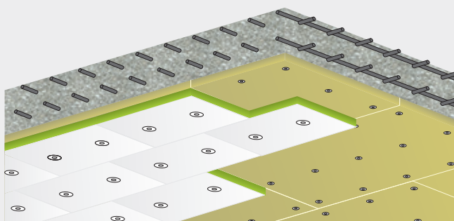
Stap 2: zeer efficiënte thermische isolatie door middel van een extra ROCKWOOL isolatieplaat
